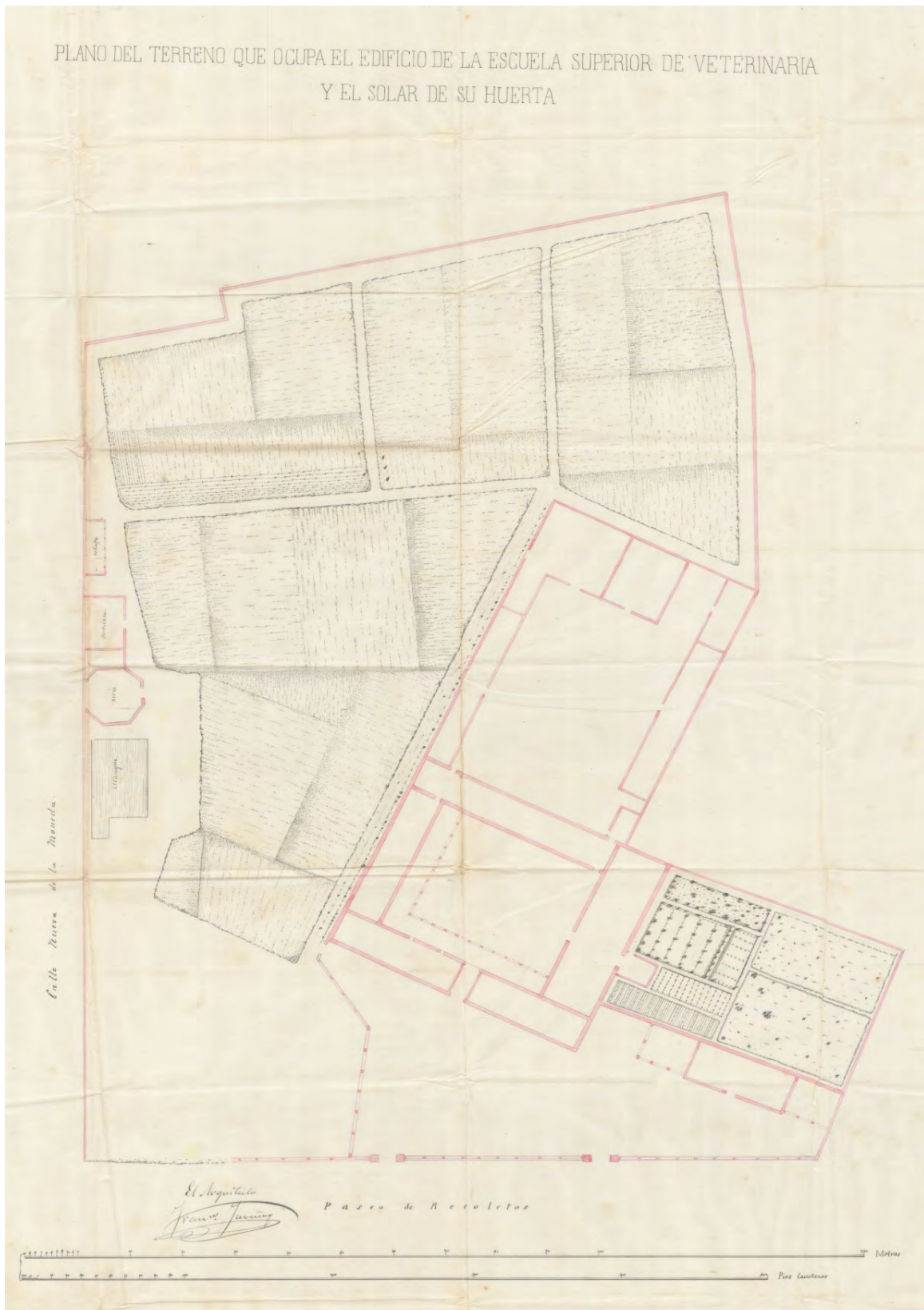
A.G.A., sección construcciones civiles, caja 31/8120, legajo 8884, expediente 3. Estado actual de la Escuela de Veterinaria. Planta Baja. Se articula el edificio, con acceso principal por el Paseo de Recoletos, en torno a dos grandes espacios interiores, señalados como patios A y B, complementado con un gran jardín, diferenciado del espacio ocupado por la huerta.
