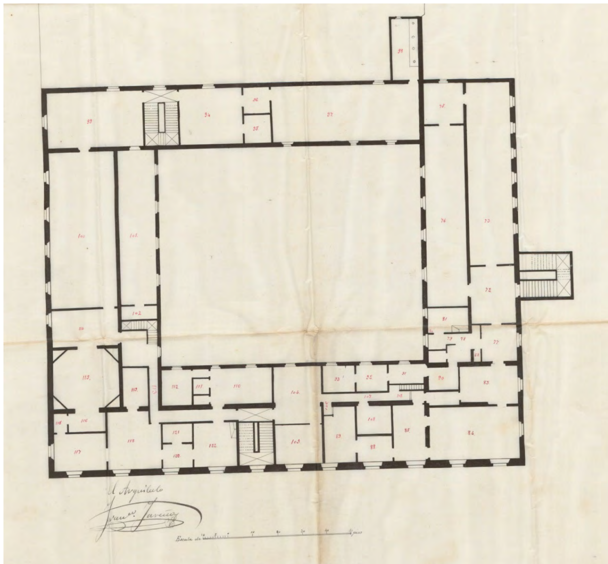
A.G.A., sección construcciones civiles, caja 31/8120, legajo 8884, expediente 3. Plano del terreno que ocupa el edificio de la Escuela Superior de Veterinaria y el solar de su huerta. Los tres planos expuestos, contienen la firma del arquitecto Francisco Jareño.
